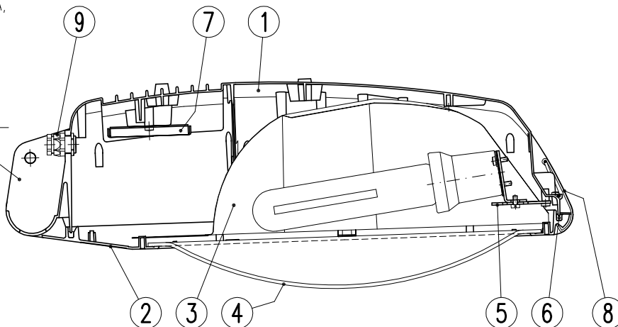
SECCION LONGITUDINAL
